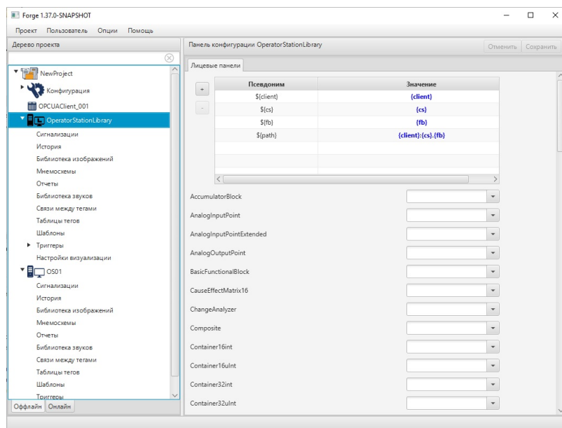
Рисунок 15. Библиотека станции оператора в дереве проекта
