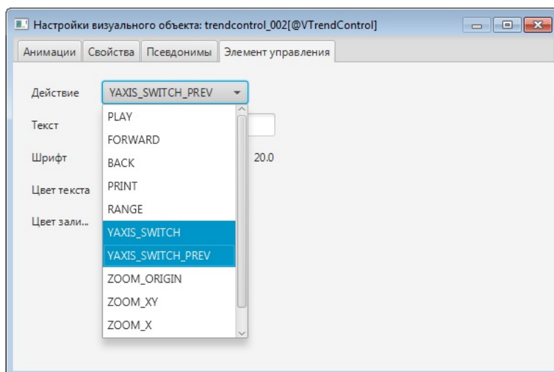
Рисунок 89. Выбор переключателя оси Y вперед/назад
