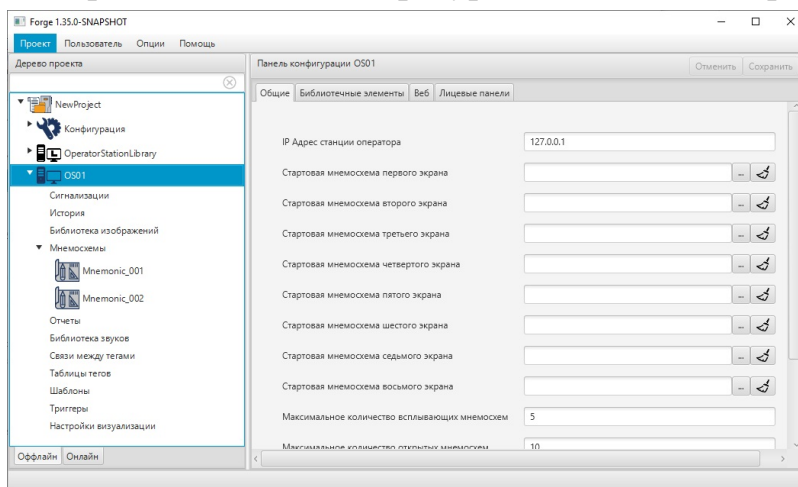
Рисунок 27. Окно управления стартовыми мнемосхемами
