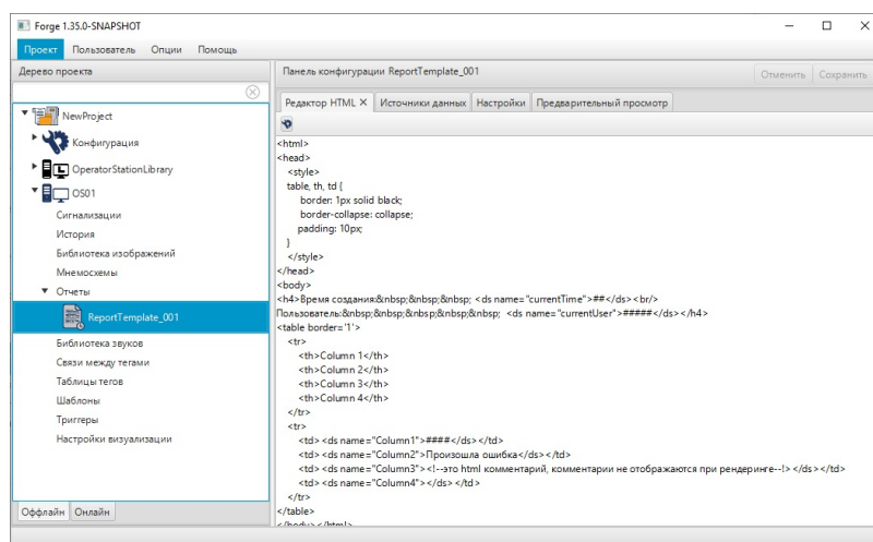
Рисунок 244. Отчет в дереве проекта
