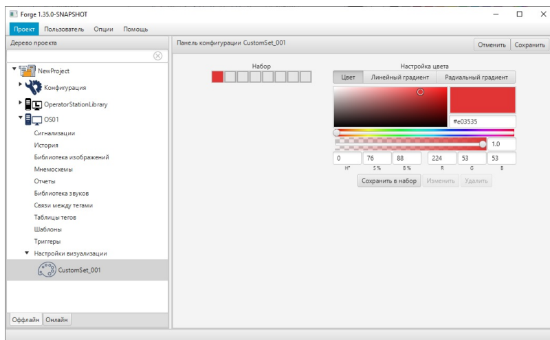
Рисунок 240. Добавление цвета в пользовательский набор
