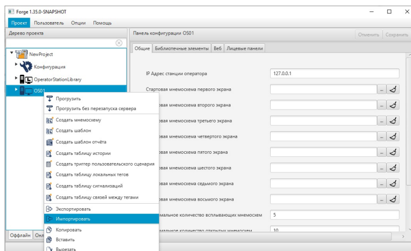
Рисунок 8. Импорт станции оператора
