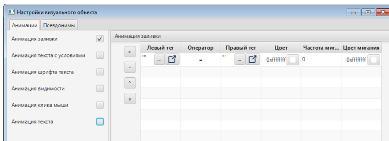
Рисунок 152. Формирование анимации заливки
