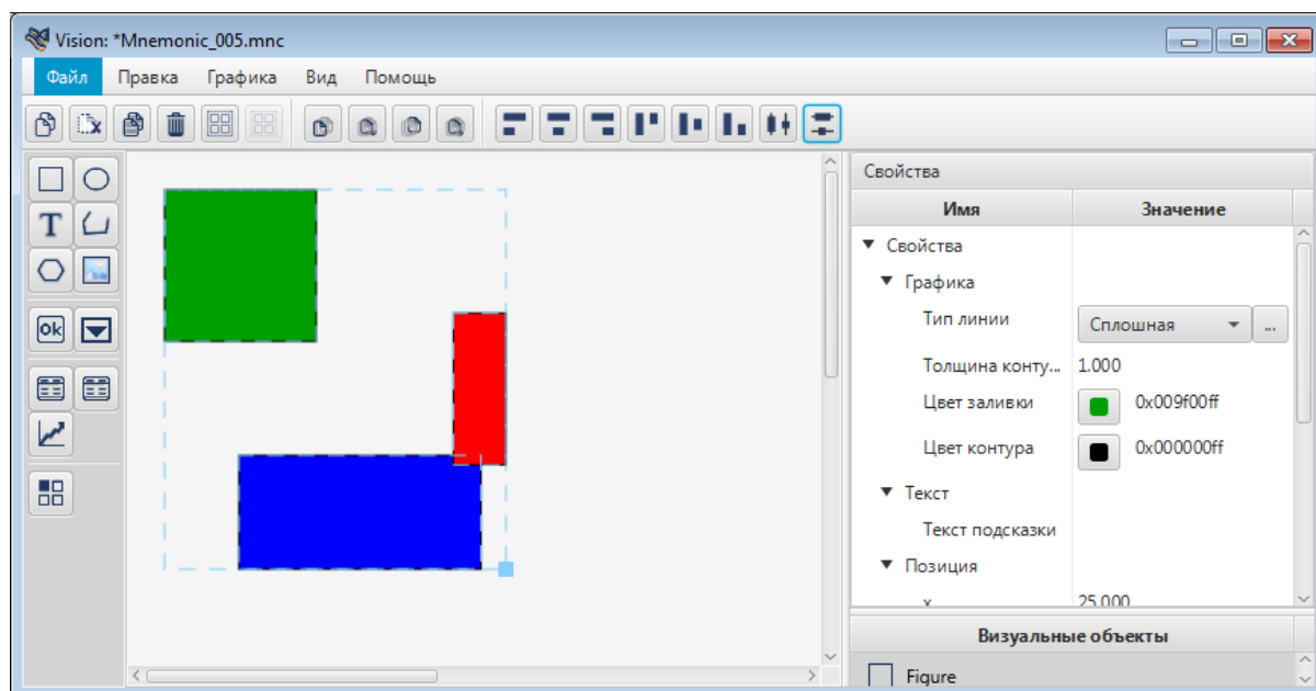
Рисунок 113. Окно редактора мнемосхем
