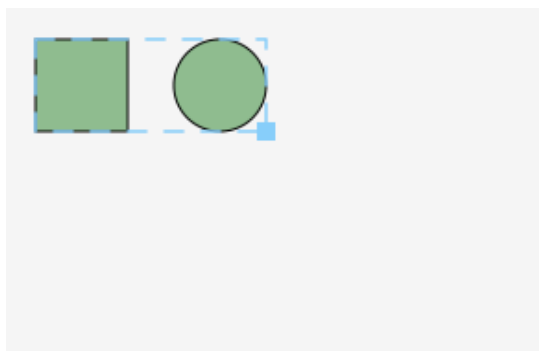
Рисунок 112. Элементы сгруппированы
