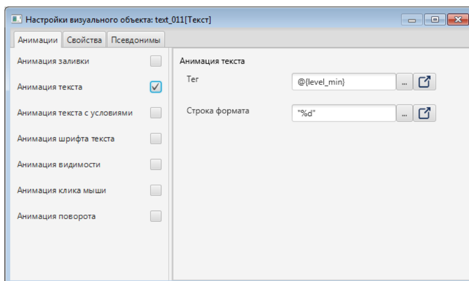
Рисунок 176. Анимация текста
