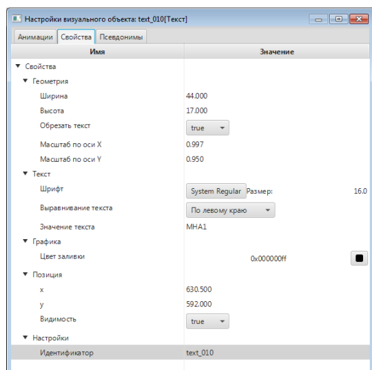
Рисунок 42. Вкладка Свойства
