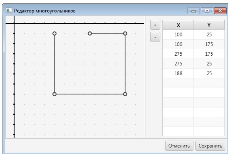
Рисунок 124. Добавление вершины
