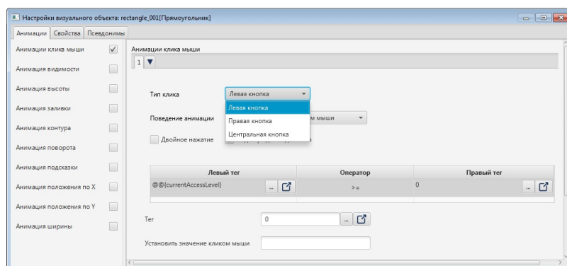
Рисунок 163. Тип клика
