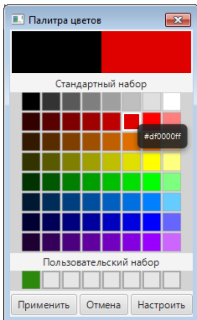
Рисунок 118. Палитра цветов
