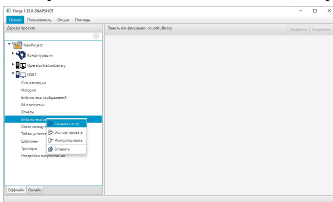
Рисунок 234. Создание папки
