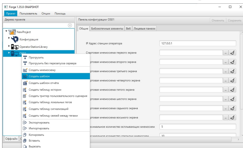
Рисунок 133. Создание шаблона
