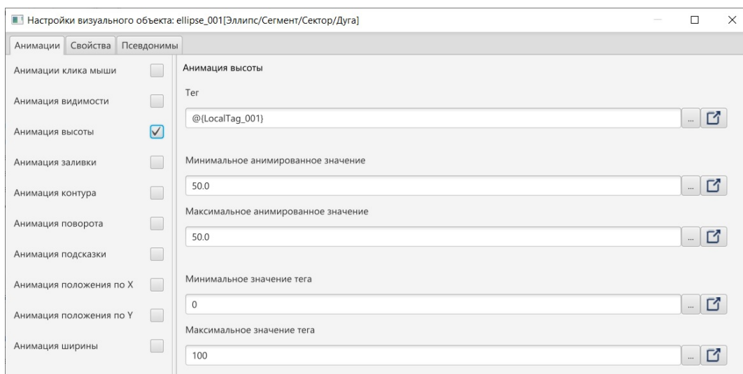
Рисунок 173. Анимация высоты
