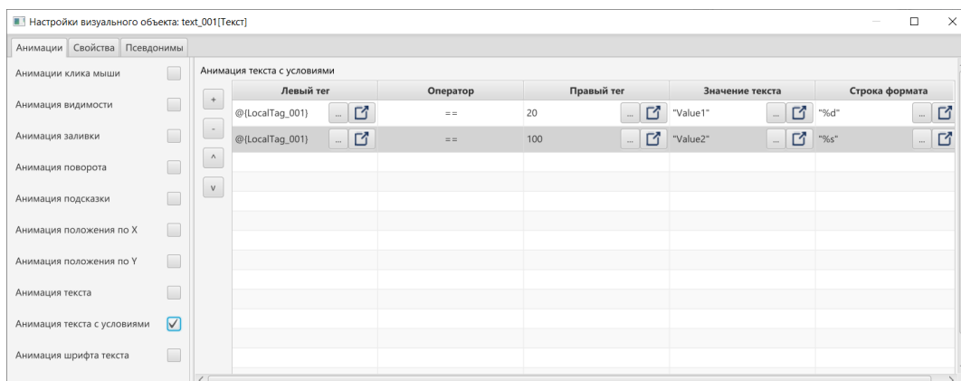
Рисунок 185. Формирование условий
