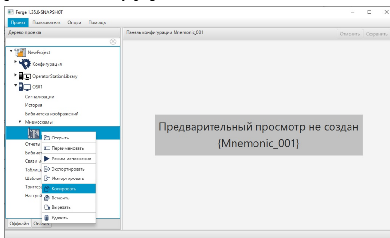
Рисунок 25. Копирование мнемосхемы
