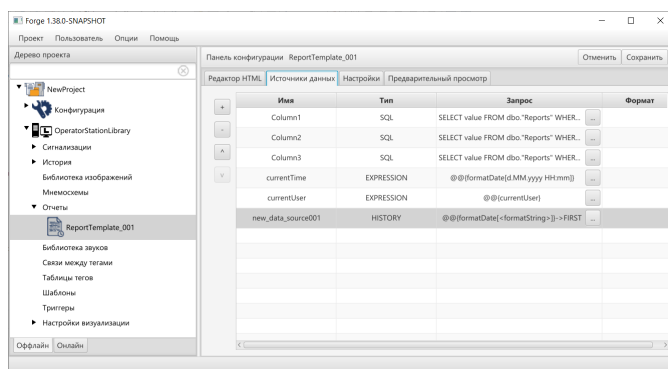
Рисунок 247. Источники данных
