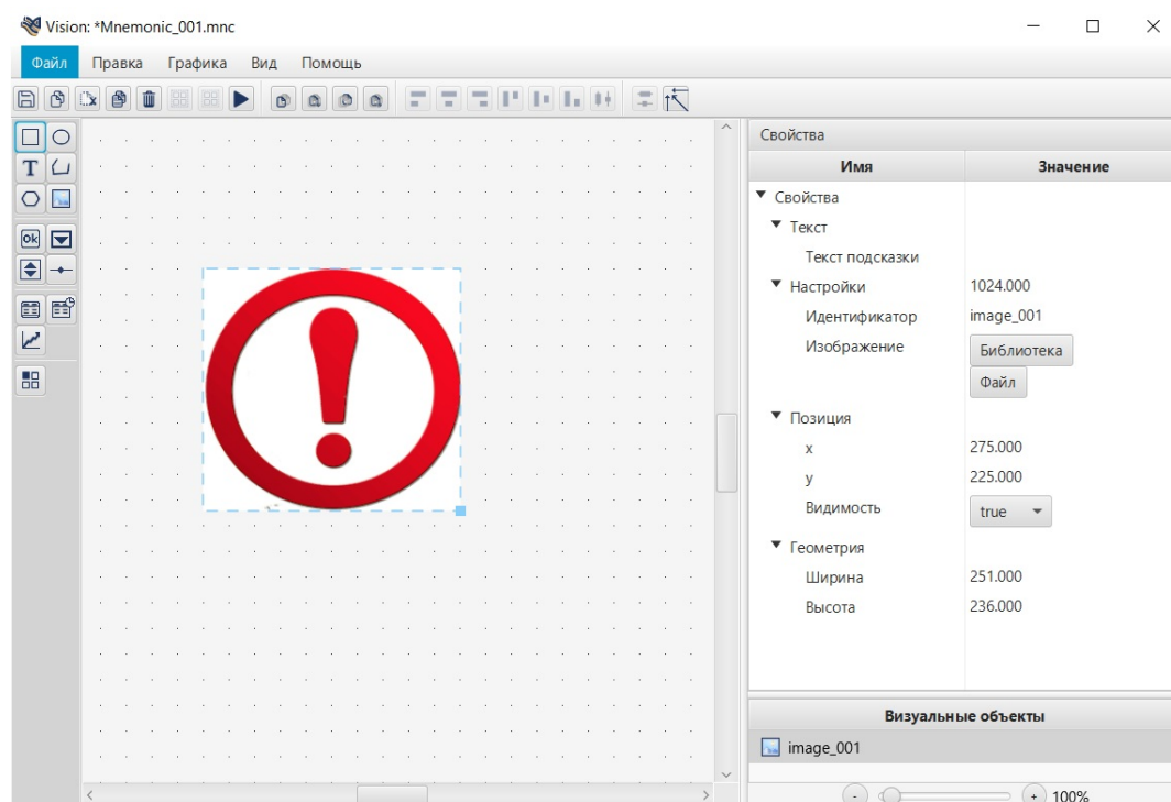
Рисунок 76. Свойства изображения
