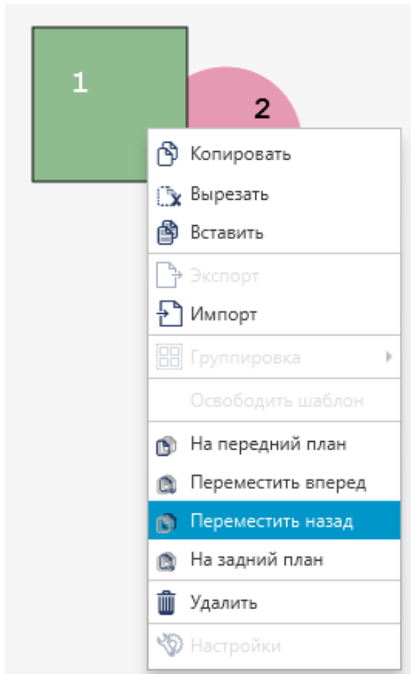
Рисунок 115. Перемещение
