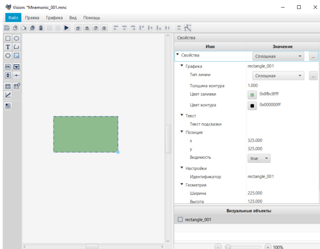
Рисунок 47. Настройка прямоугольника
