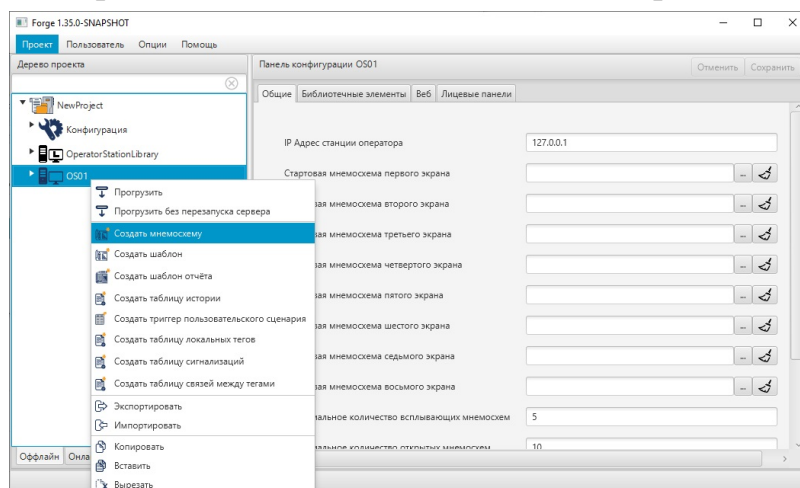
Рисунок 16. Создание мнемосхемы
