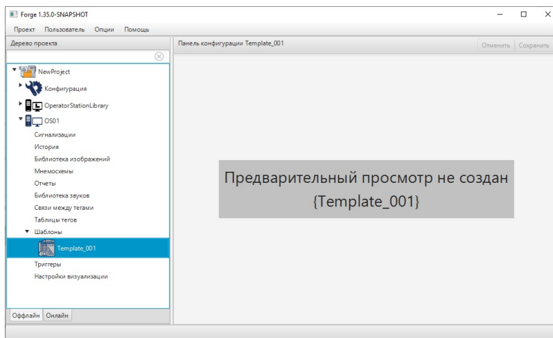
Рисунок 135. Открытие шаблона
