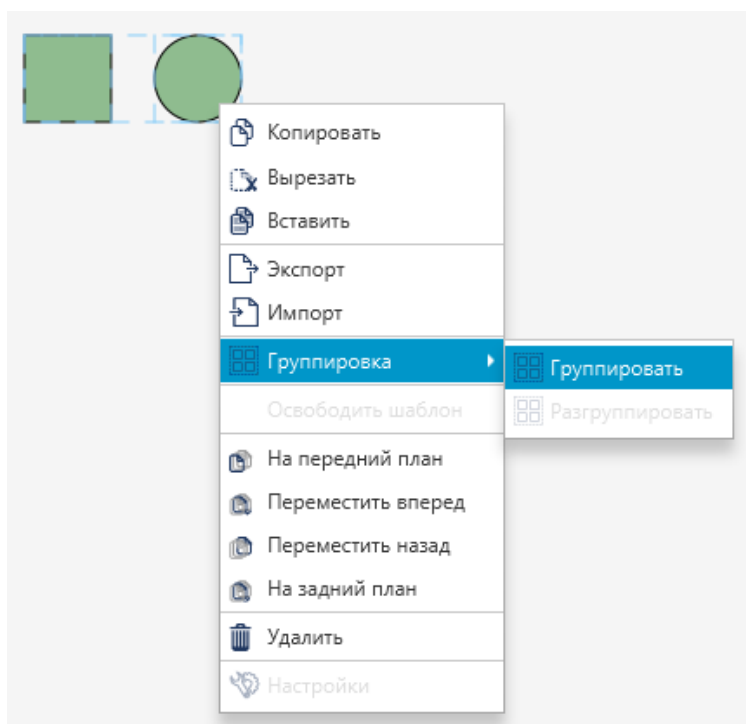
Рисунок 111. Группировка
