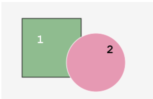
Рисунок 116. Объект перемещен
