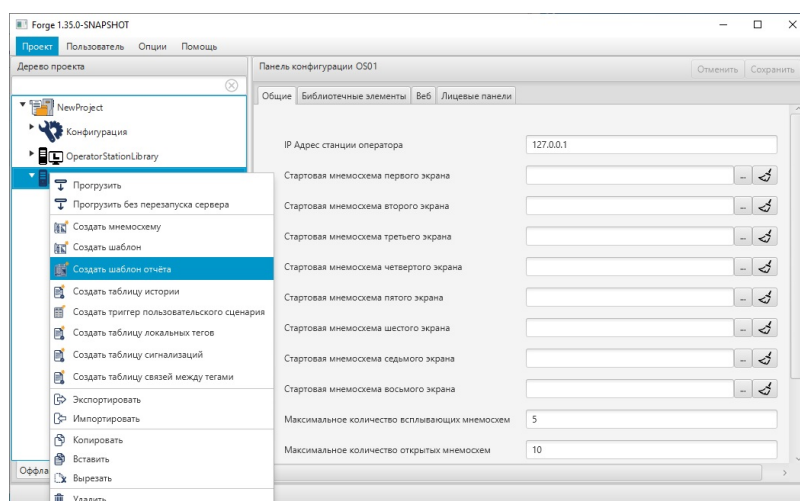
Рисунок 243. Создание отчета
