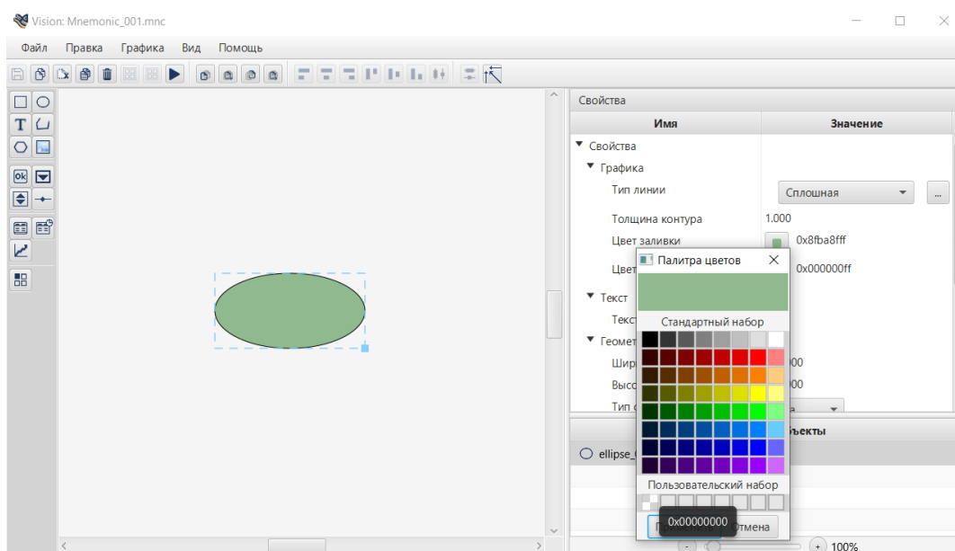
Рисунок 58. Настройка прозрачности
