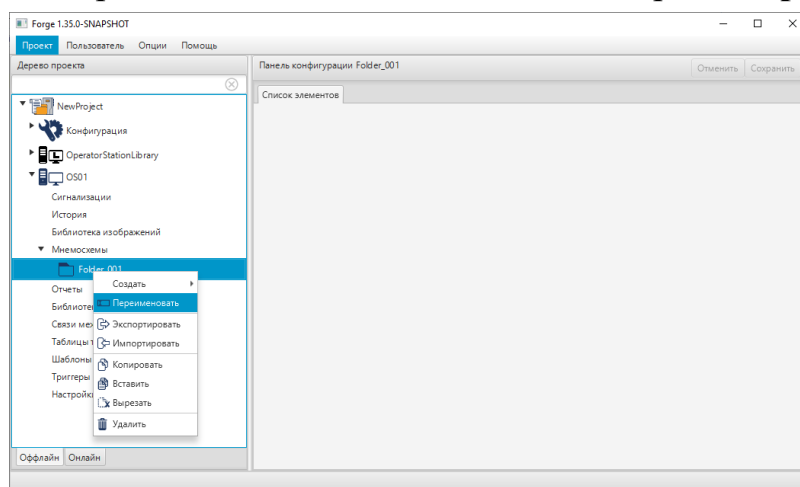
Рисунок 33. Переименование папки
