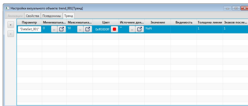
Рисунок 82. Настройка тренда
