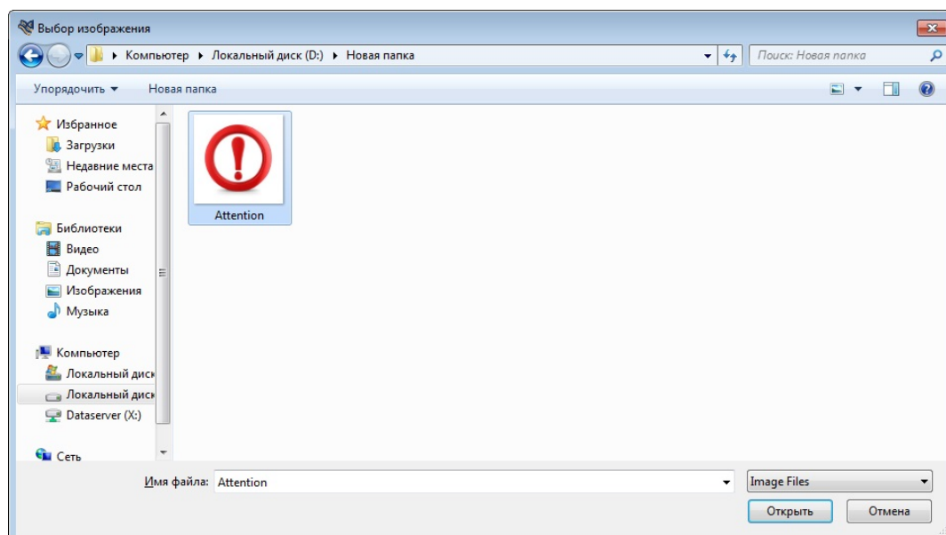
Рисунок 75. Выбор изображения
