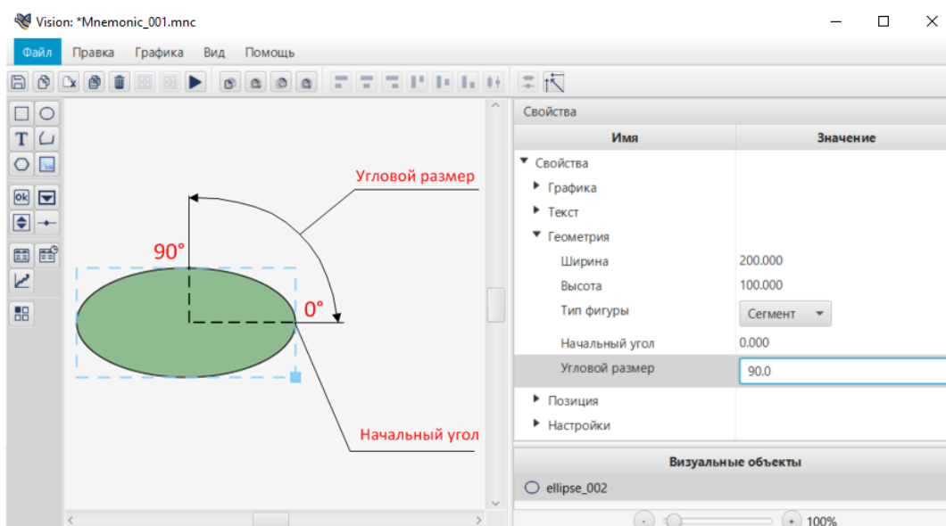
Рисунок 55. Настройка сегмента
