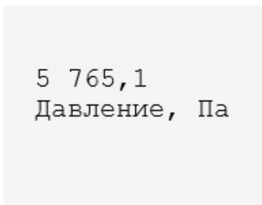
Рисунок 179. Пример 3
