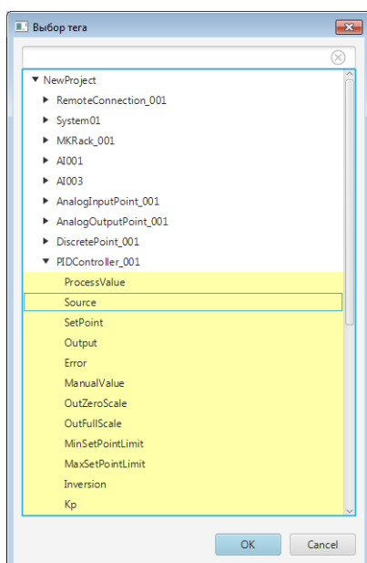
Рисунок 214. Выбор тега
