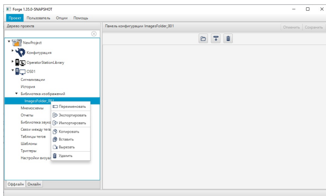
Рисунок 233. Операции с папкой в библиотеке изображений
