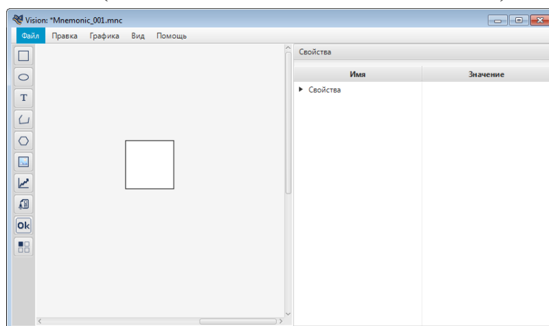
Рисунок 153. Формирование анимации заливки
