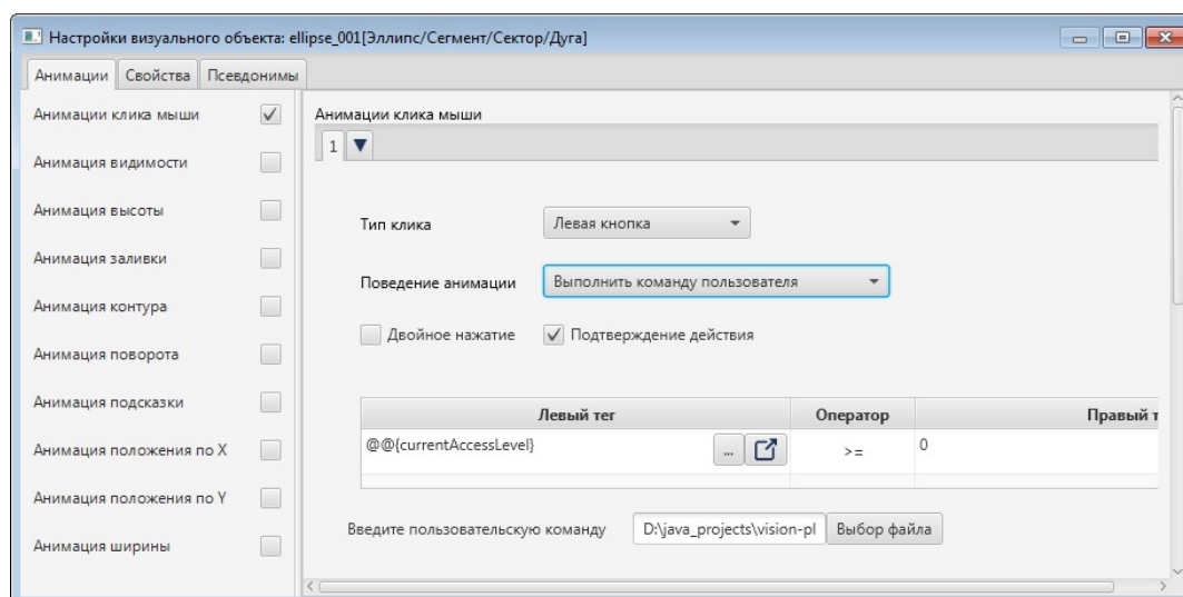
Рисунок 172. Анимация клика мыши. Выполнение команды пользователя
