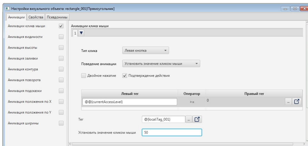
Рисунок 166. Анимация клика мыши. Установление значения кликом мыши
