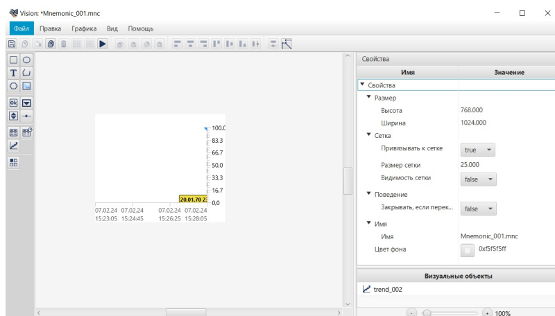
Рисунок 81. Тип объекта - тренд
