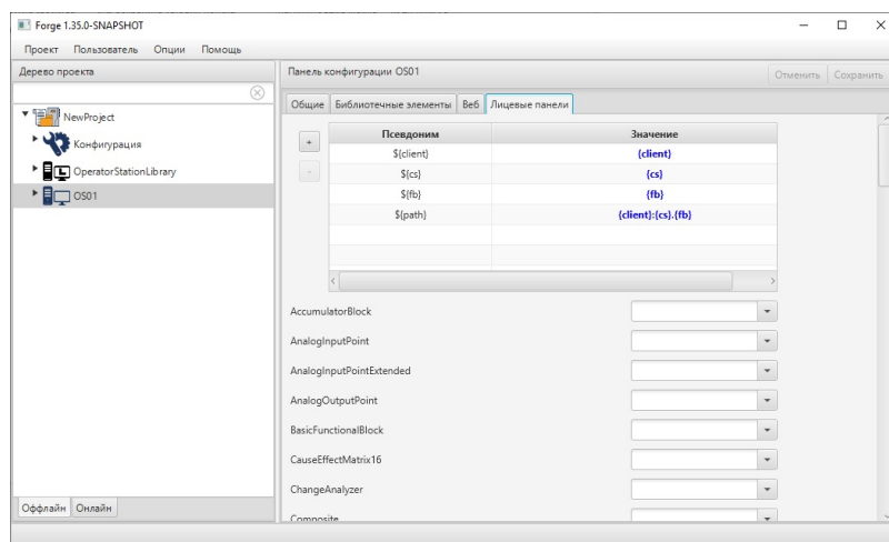
Рисунок 14. Привязка лицевой панели
