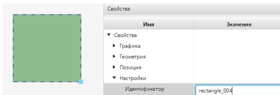
Рисунок 117. Переименование идентификатора
