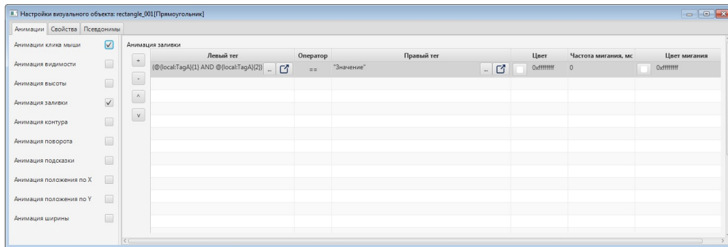
Рисунок 132. Применение выражений
