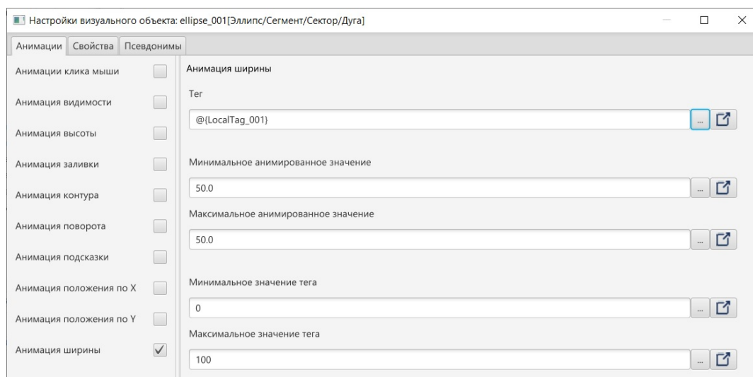
Рисунок 174. Анимация ширины
