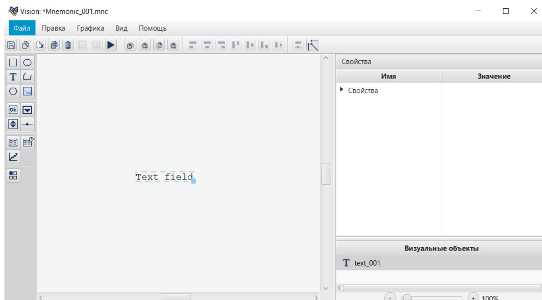
Рисунок 61. Текст
