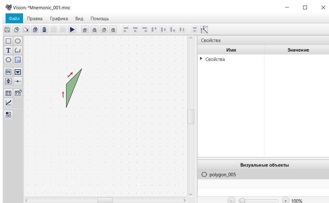
Рисунок 71. Построение многоугольника
