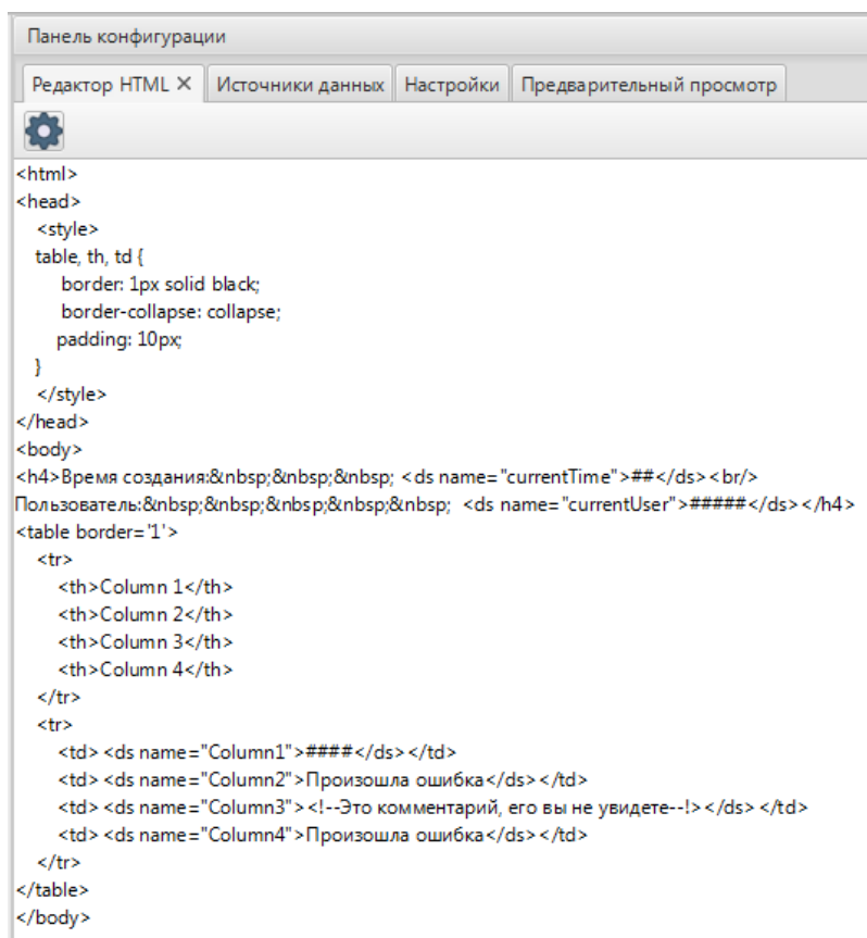
Рисунок 249. Редактор HTML
