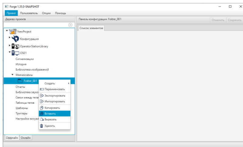
Рисунок 35. Вставка папки
