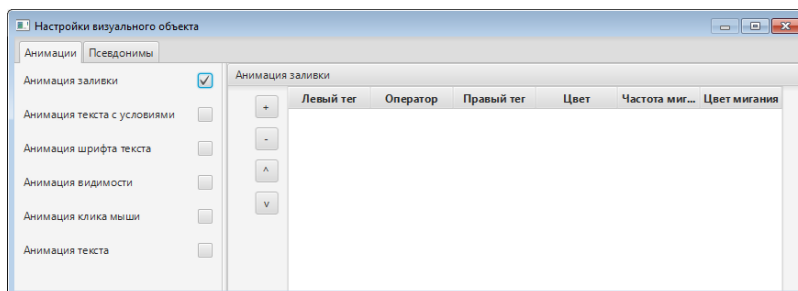
Рисунок 151. Анимация заливки
