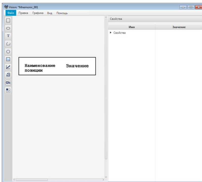
Рисунок 143. Добавление шаблона
