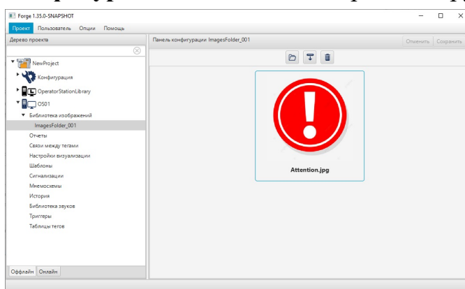
Рисунок 231. Панель конфигурации
