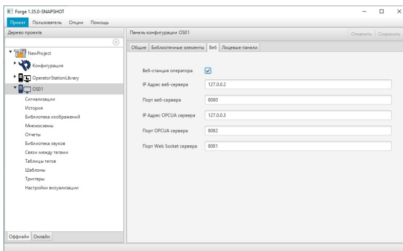
Рисунок 5. Вкладка "Веб"
