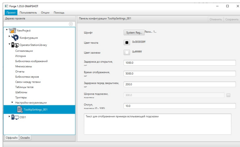
Рисунок 239. Настройка подсказки
