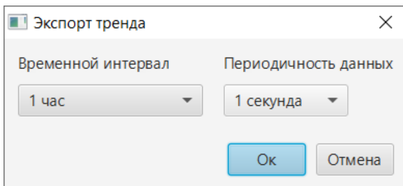
Рисунок 92. Экспорт тренда
