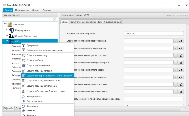
Рисунок 226. Создание триггера
