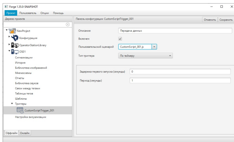
Рисунок 228. Настройка триггера
