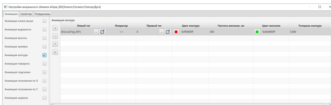
Рисунок 175. Анимация контура
