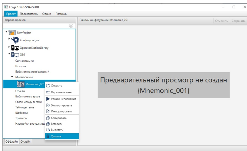
Рисунок 26. Удаление мнемосхемы
