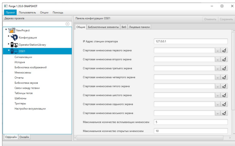
Рисунок 3. Вкладка "Общие"
