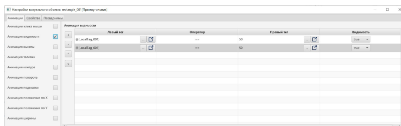
Рисунок 159. Анимация видимости
