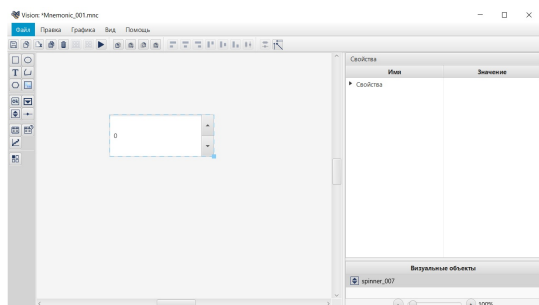
Рисунок 100. Счётчик
