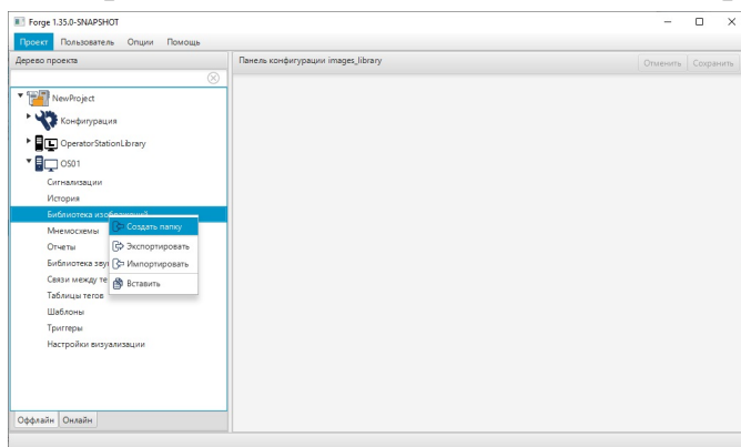
Рисунок 229. Создание папки
