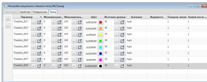
Рисунок 84. Настройка тренда
