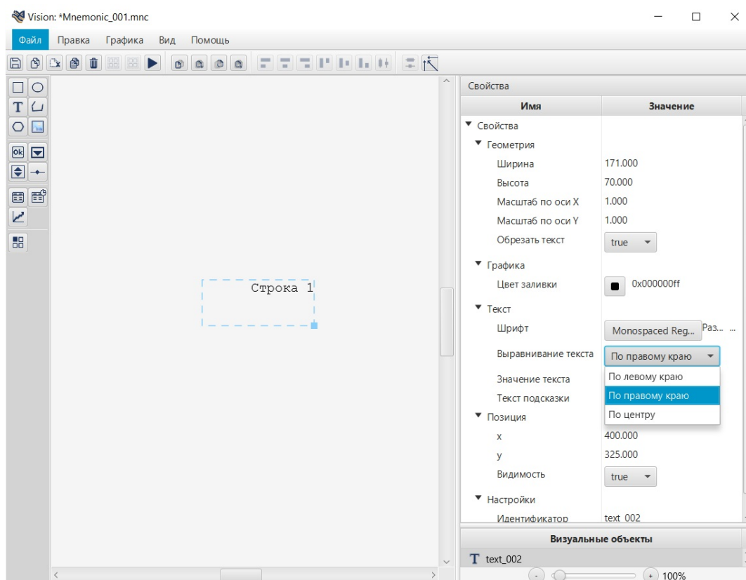
Рисунок 64. Выравнивание текста
