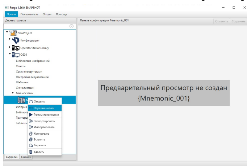
Рисунок 18. Переименование мнемосхемы
