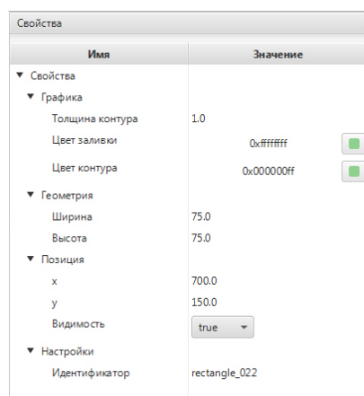
Рисунок 40. Окно свойств
