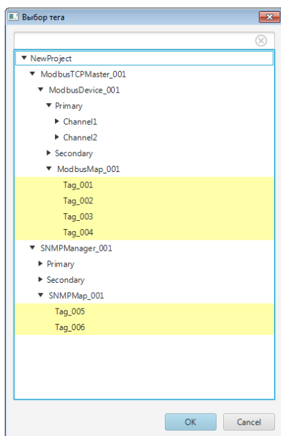
Рисунок 210. Выбор атрибута
