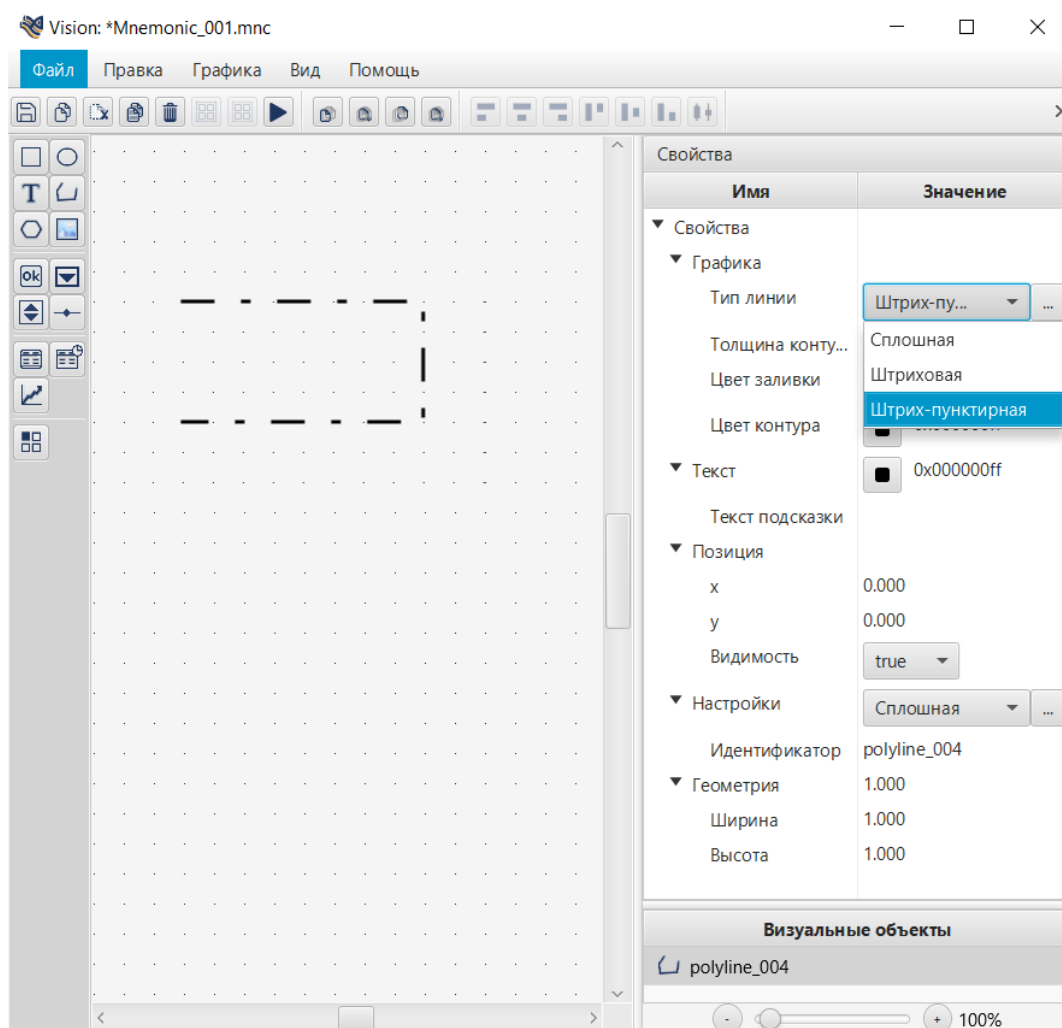
Рисунок 68. Настройка ломаной
