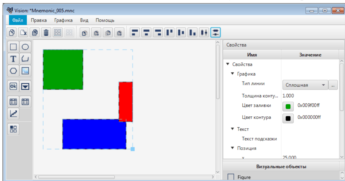
Рисунок 104. Панель операций
