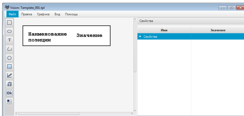
Рисунок 136. Построение шаблона
