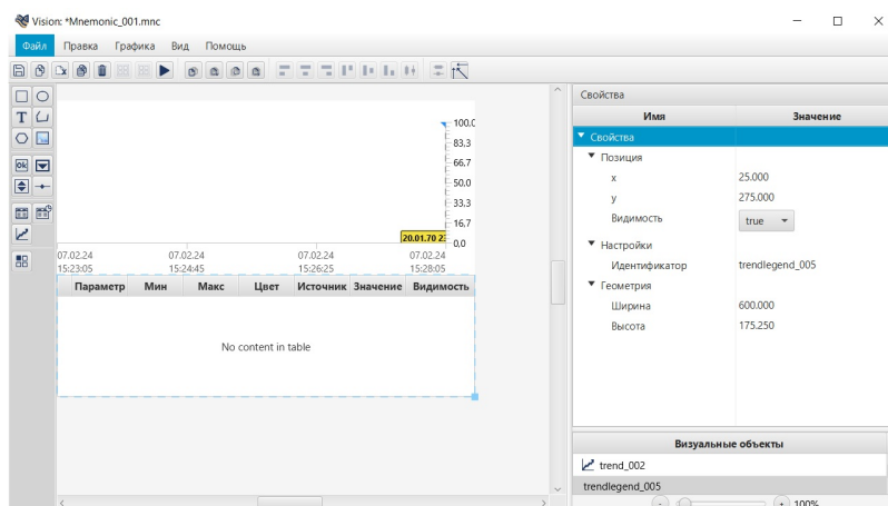
Рисунок 94. Настройка легенды
