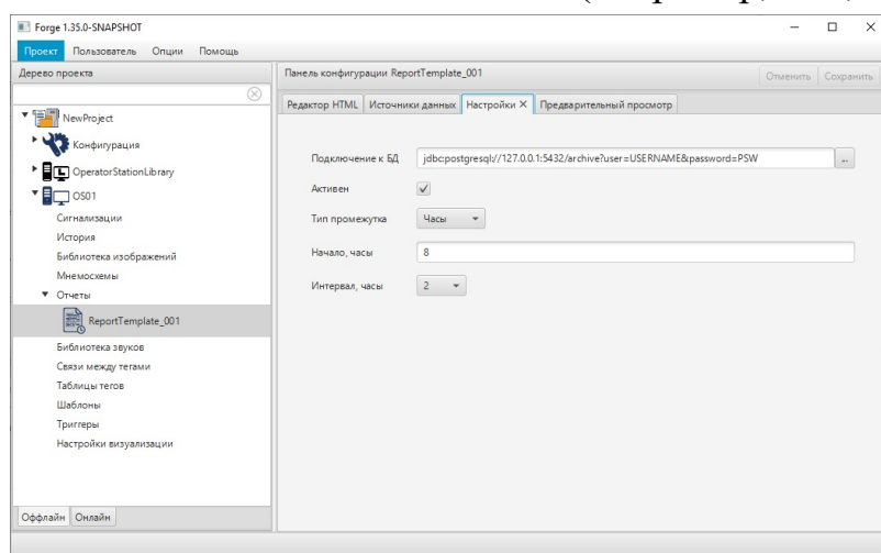
Рисунок 245. Настройка отчета
