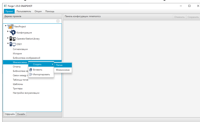
Рисунок 30. Создание папки
