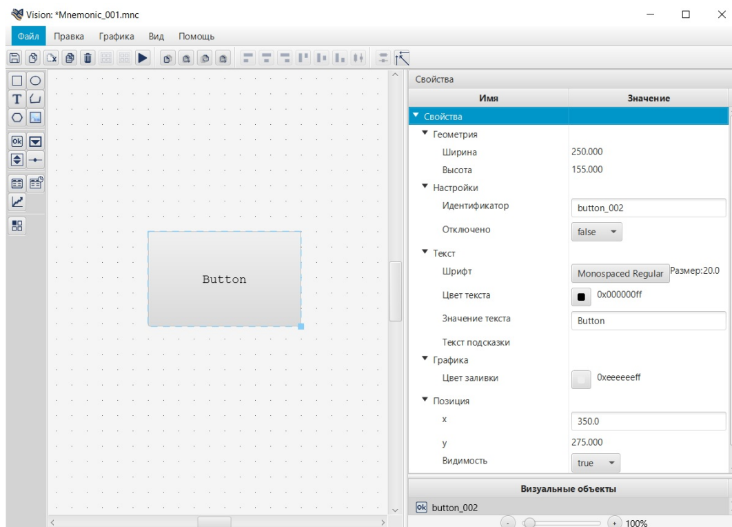
Рисунок 78. Настройка кнопки
