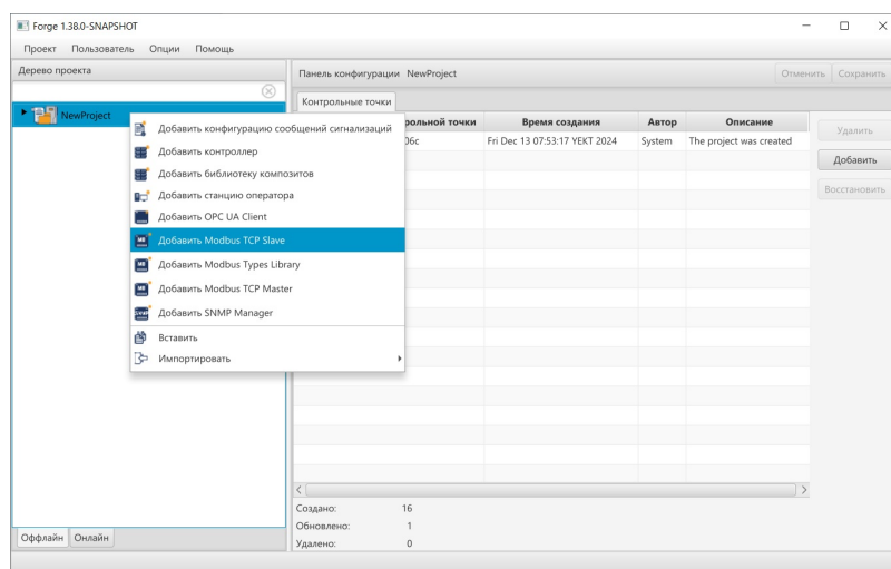
Рисунок 1. Добавление Modbus TCP Slave
