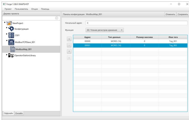
Рисунок 16. Карта Modbus в дереве проекта
