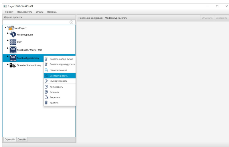
Рисунок 21. Экспорт Modbus Types Library
