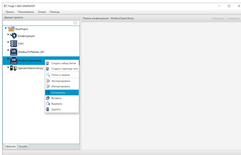
Рисунок 23. Копирование Modbus Types Library
