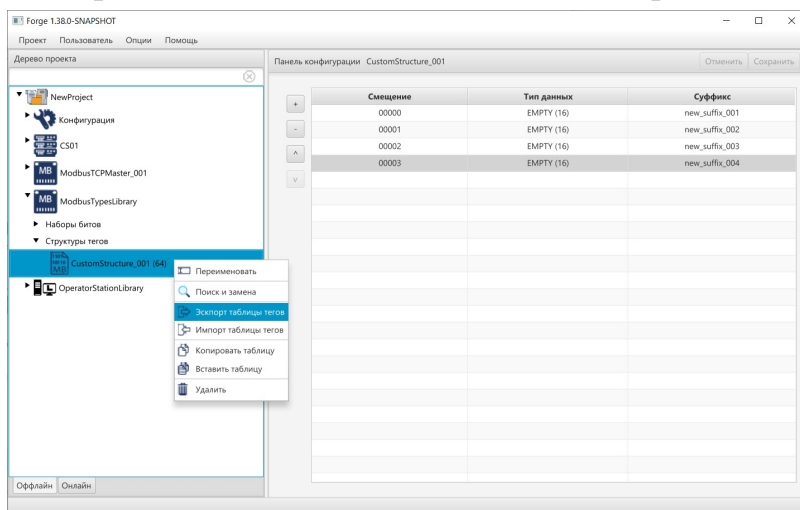
Рисунок 41. Экспорт таблицы структуры тега
