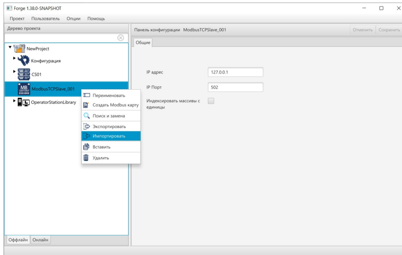
Рисунок 5. Импорт Modbus TCP Slave
