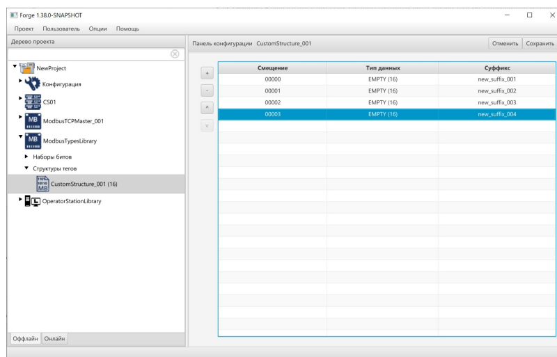
Рисунок 36. Настройка структуры тега
