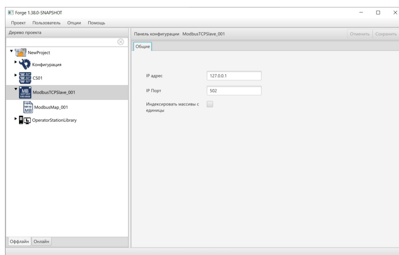
Рисунок 13. Настройка Modbus TCP Slave
