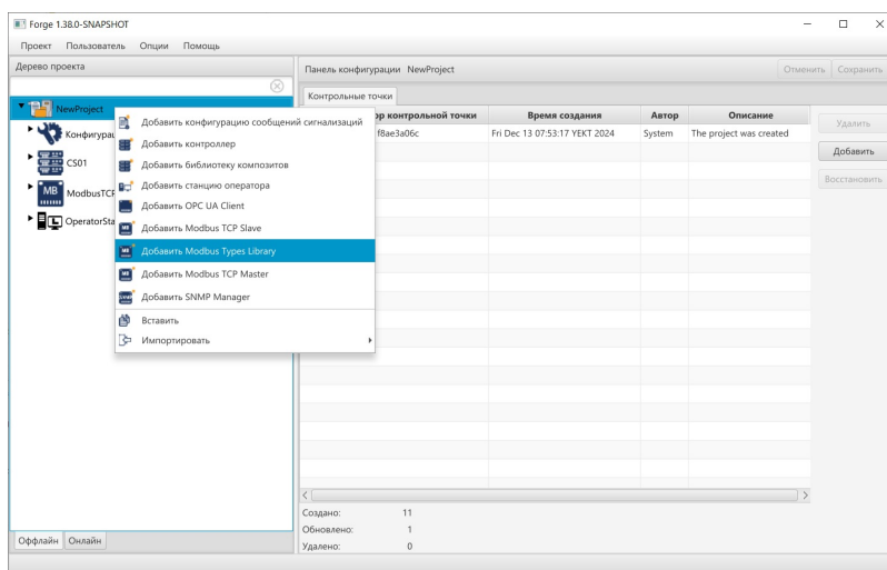
Рисунок 18. Добавление библиотеки типов Modbus
