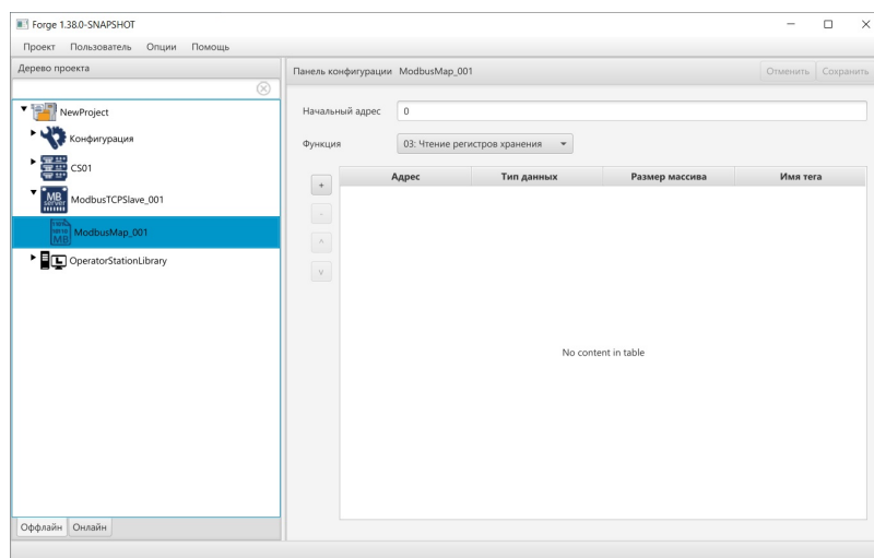
Рисунок 10. Карта Modbus TCP Slave в дереве проекта
