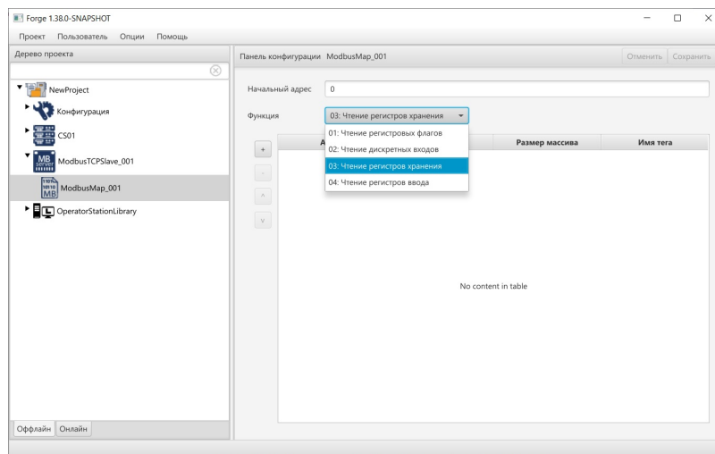
Рисунок 15. Настройка карты Modbus
