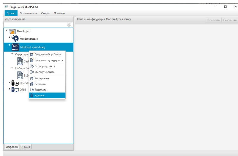
Рисунок 44. Удаление Modbus Types Library
