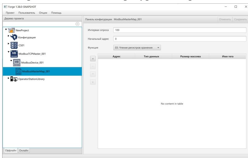
Рисунок 22. Настройка карты Modbus
