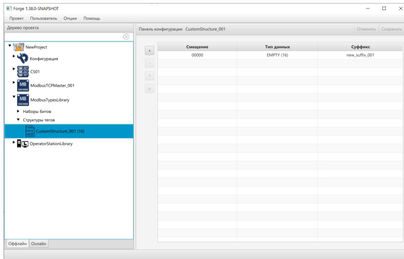
Рисунок 42. Новая структура тега в дереве проекта
