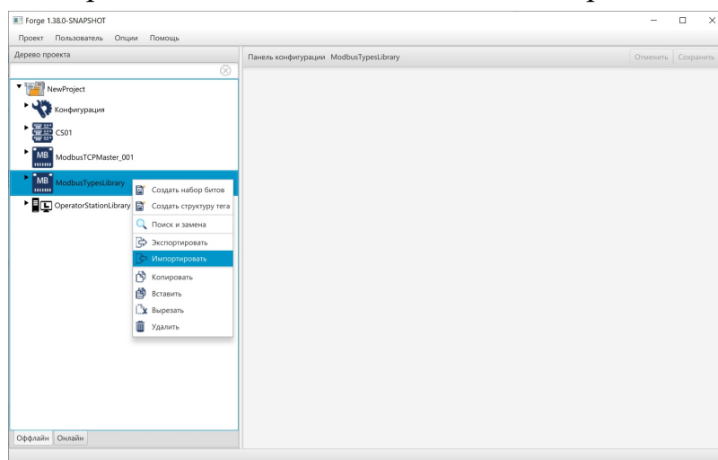
Рисунок 26. Импорт Modbus Types Library
