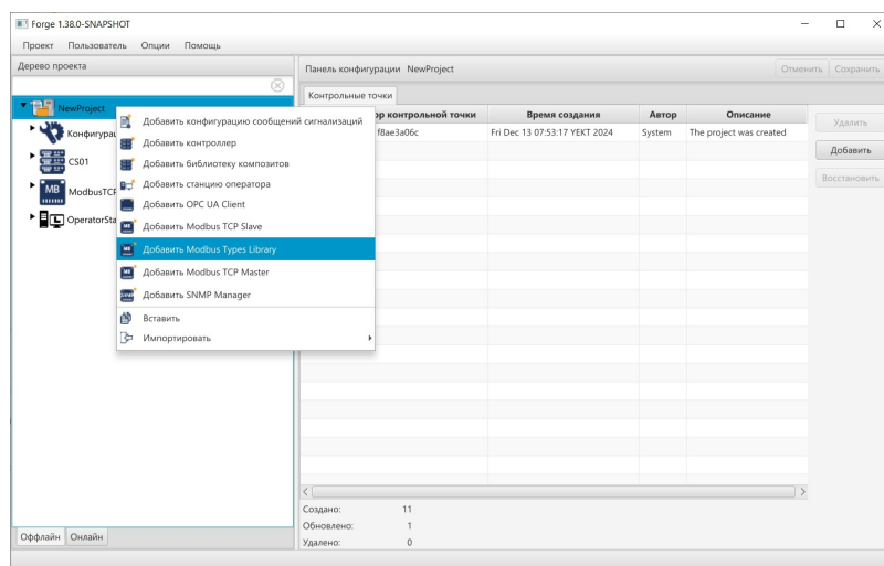
Рисунок 25. Добавление библиотеки типов Modbus
