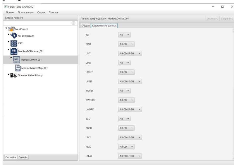
Рисунок 20. Вкладка "Кодирование данных" устройства Modbus
